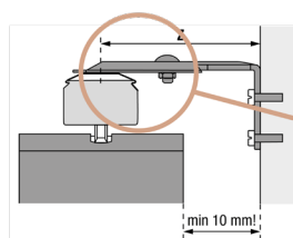
Väggmontering
