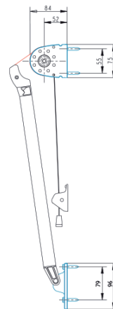
Väggmonterad DA22
