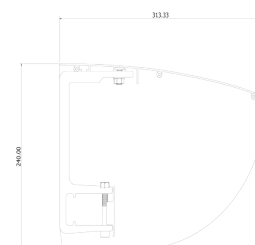
Takmontering med skyddstak
