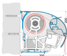
Väggmontering (mm)
