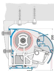
Takmontering (mm)
