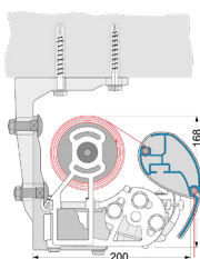
Takmontering öppen kassett (mm)
