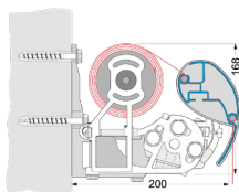
Väggmontering öppen kassett (mm)
